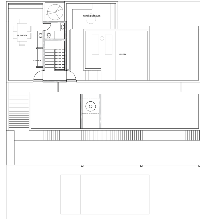
PLANTA TERRAZA esc: 1:100
