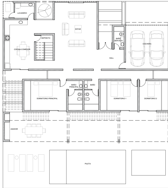
PLANTA BAJA esc: 1:100
